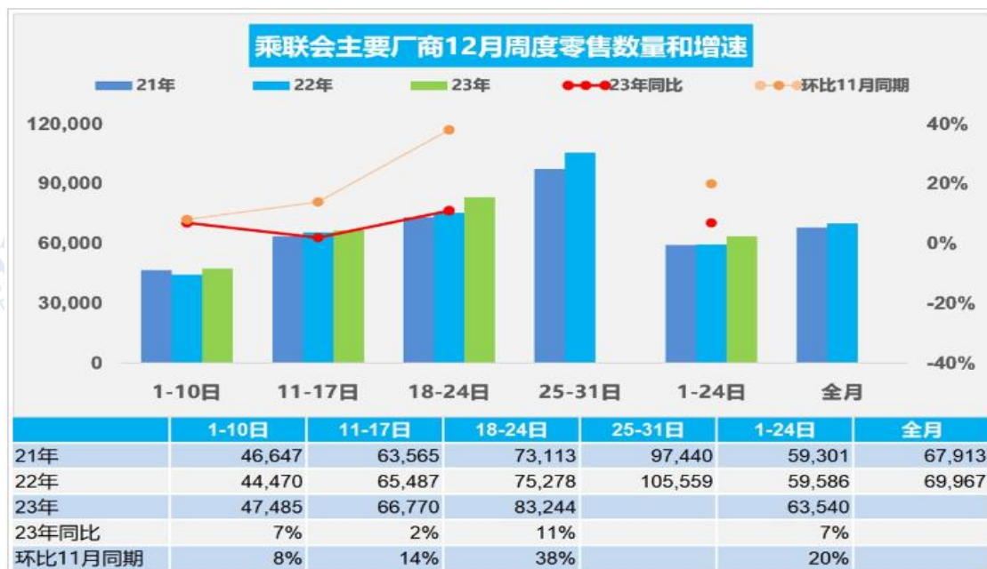
图 13: 乘用车零售
