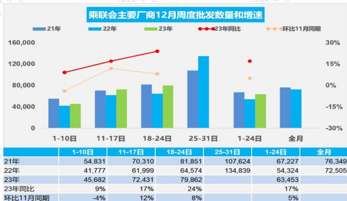
图 14: 乘用车批发
