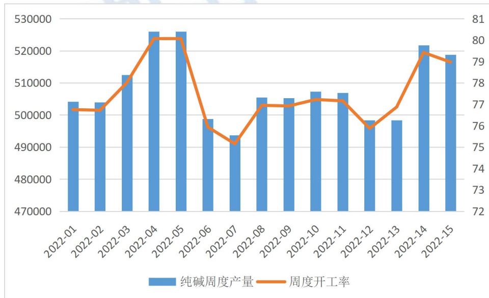
图 3：纯碱周度产量/开工率
