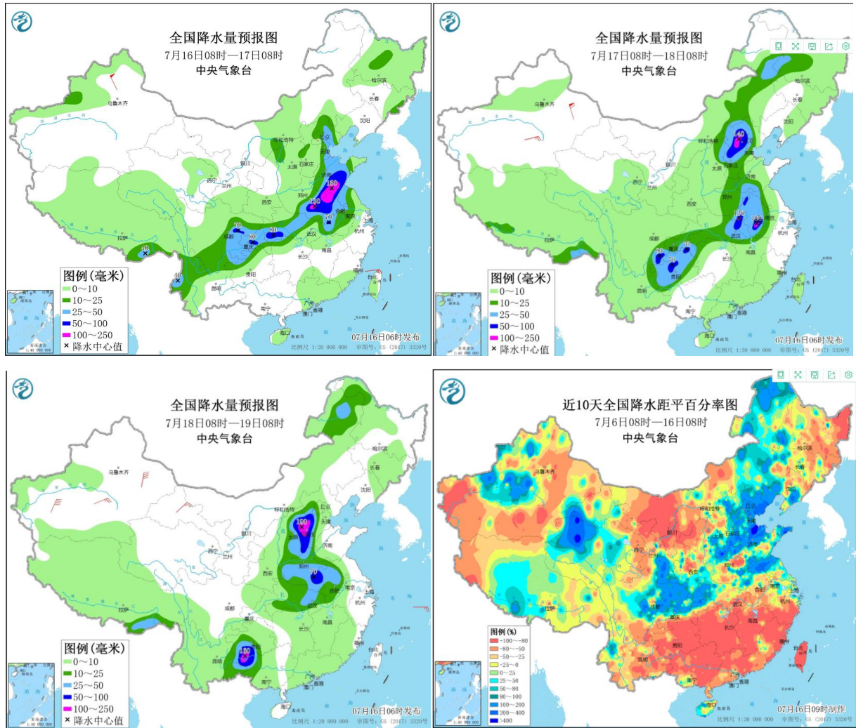
图7 全国降水量预报图 数据来源 中央气象台 和合期货
